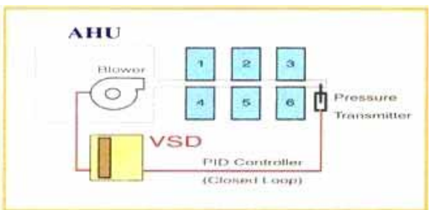
แผนภูมิแสดงการใช้กำลังงานของพัดลม/ปั๊ม
